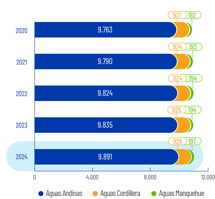
LONGITUD DE LA RED DE RECOLECCIÓN (KM)
