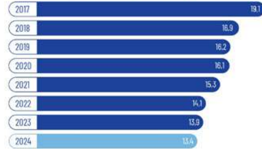
TASA DE ROTURAS CADA 100 KM EN RED DE AGUA POTABLE, GRUPO AGUAS
