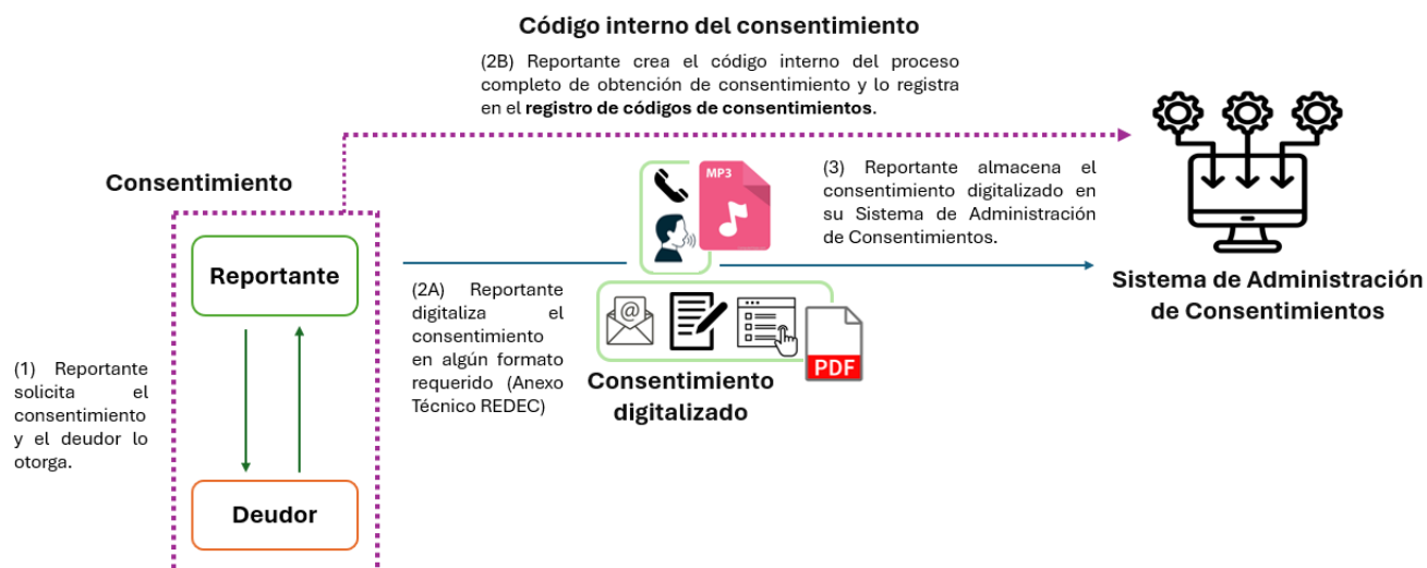
Figura 4: Codificación del consentimiento y almacenamiento en el registro de códigos de consentimientos
